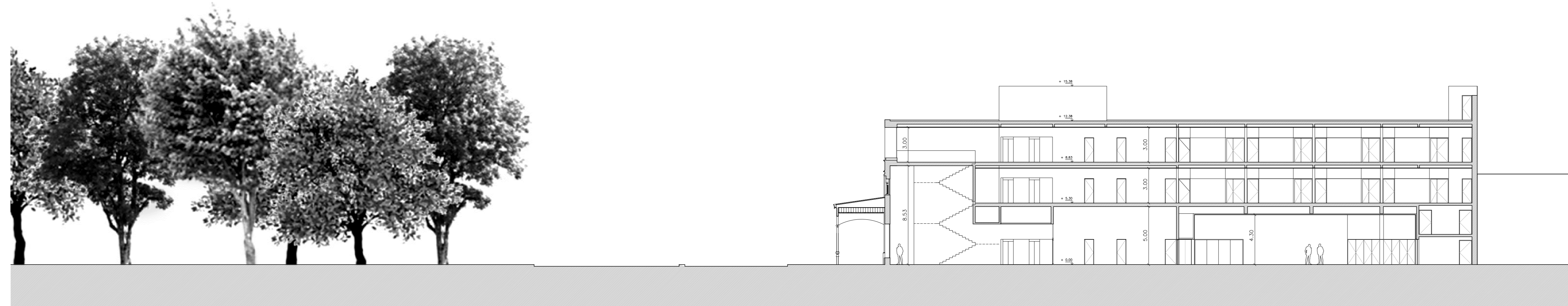
CORTE LONGITUDINAL A-A ESC.:1:200.
