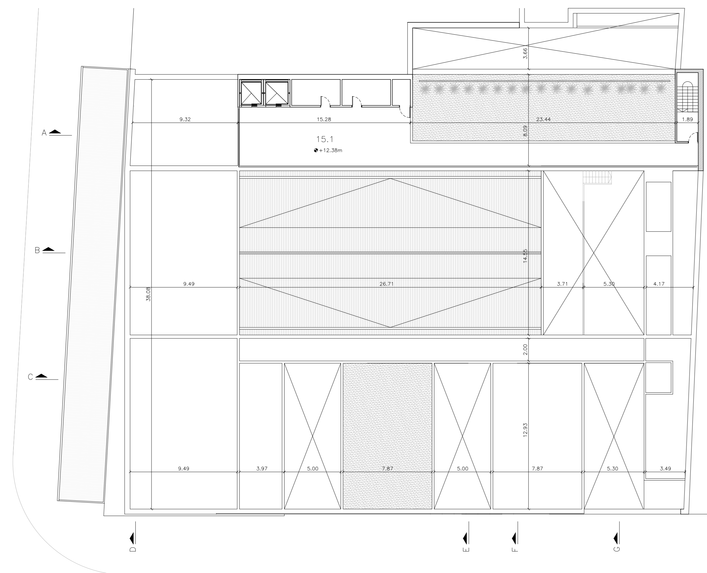
PLANTA TECHO +12.38m-ESC.:1:200.
