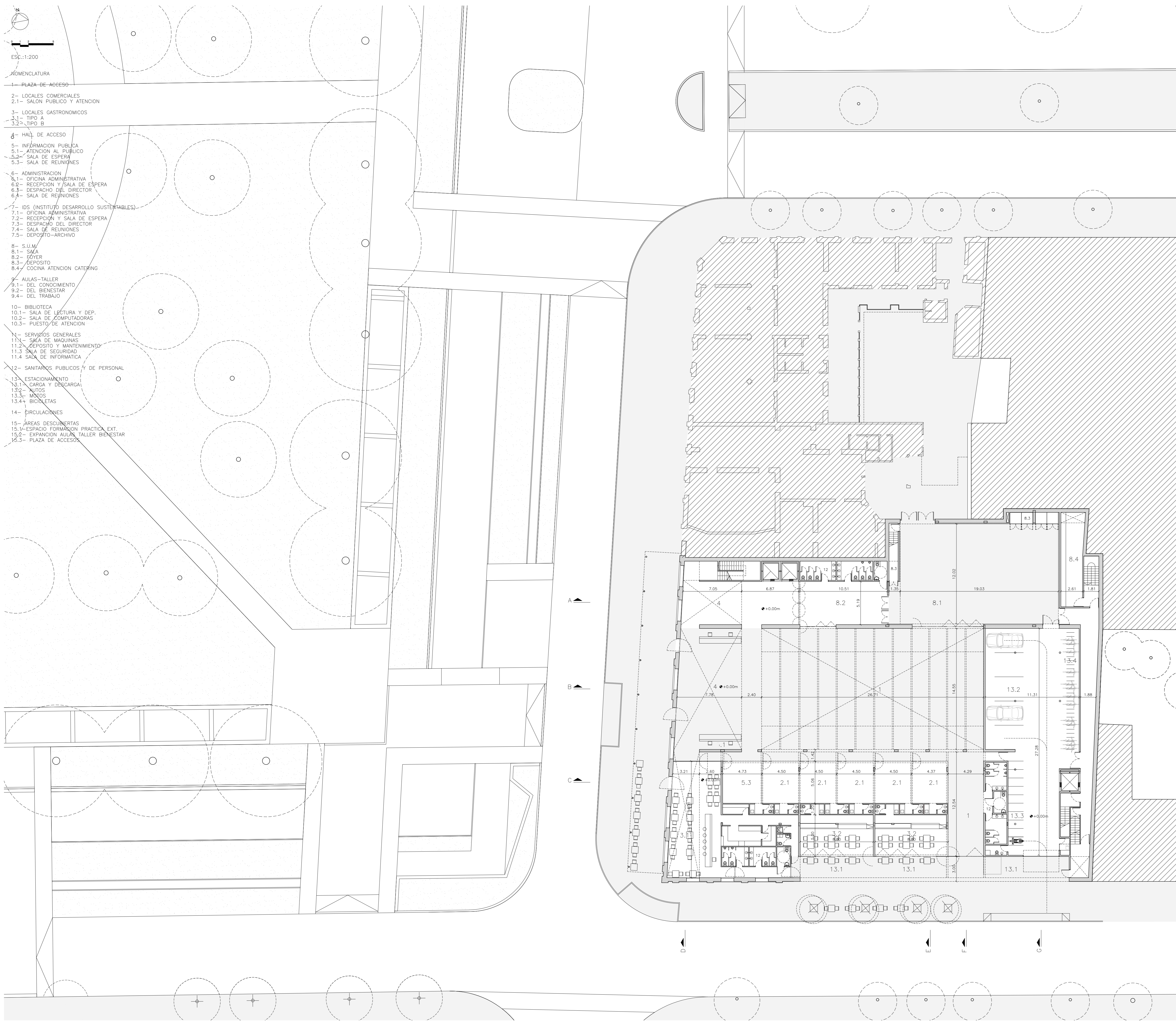
PLANTA BAJA NIVEL 0.00m ESC. 1:200
