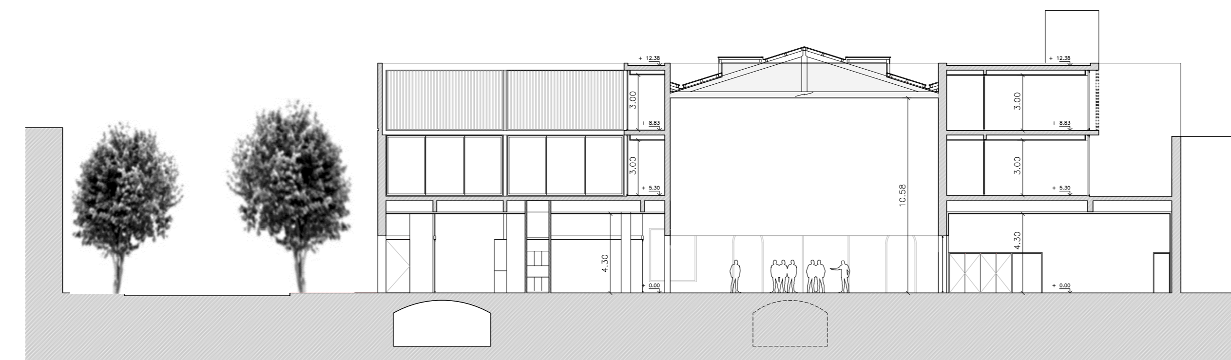
CORTE TRANSVERSAL E-E ESC.:1:200.
