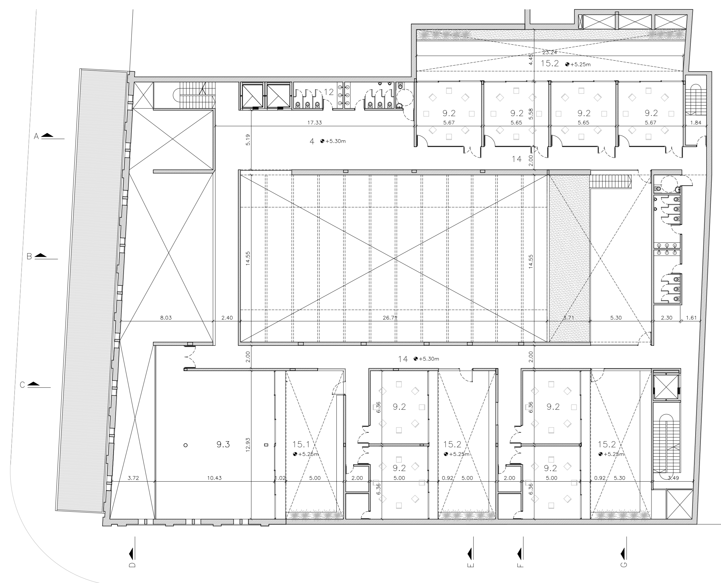
PLANTA 2do NIVEL +5.30m-ESC.:1:200.
