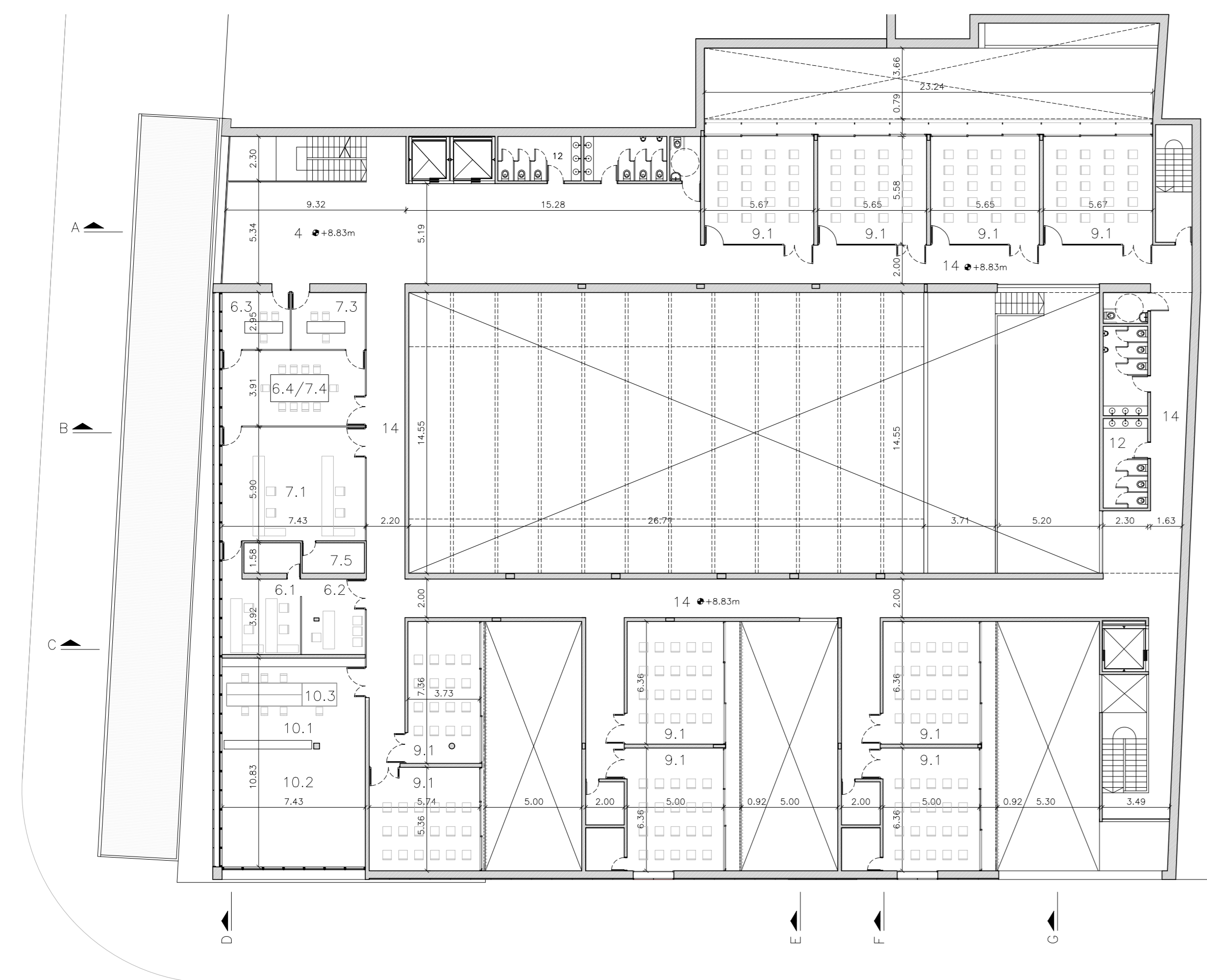
PLANTA 3er NIVEL +8.83m-ESC.:1:200.
