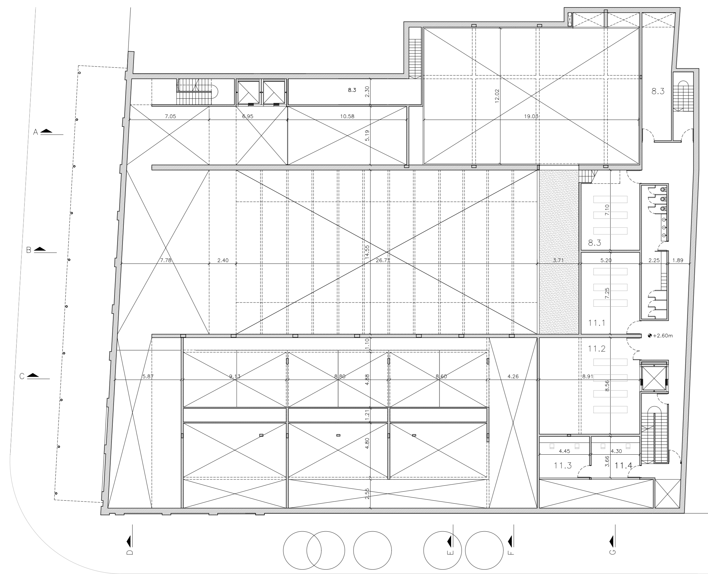
PLANTA ENTREPISO NIVEL +2.60m-ESC.:1:200.
