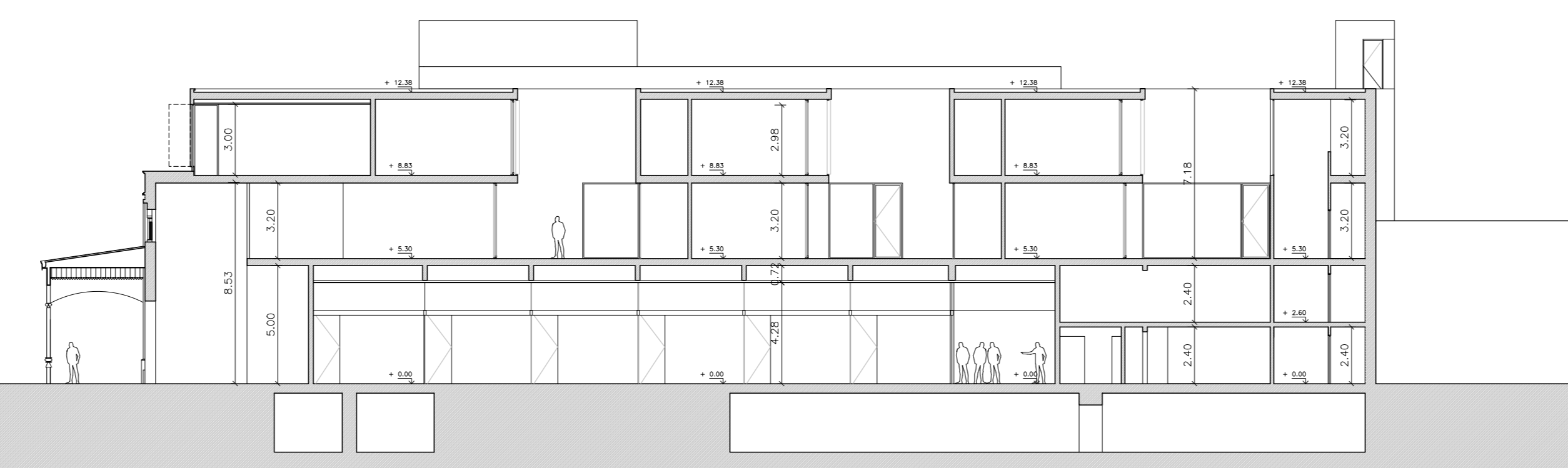
CORTE LONGITUDINAL C-C ESC.:1:200.
