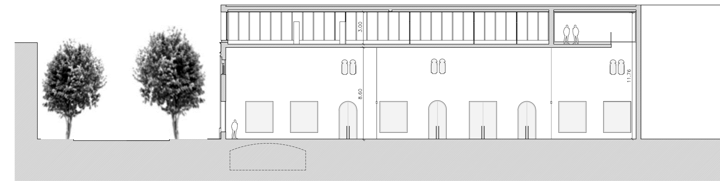
CORTE TRANSVERSAL D-D ESC.:1:200.
