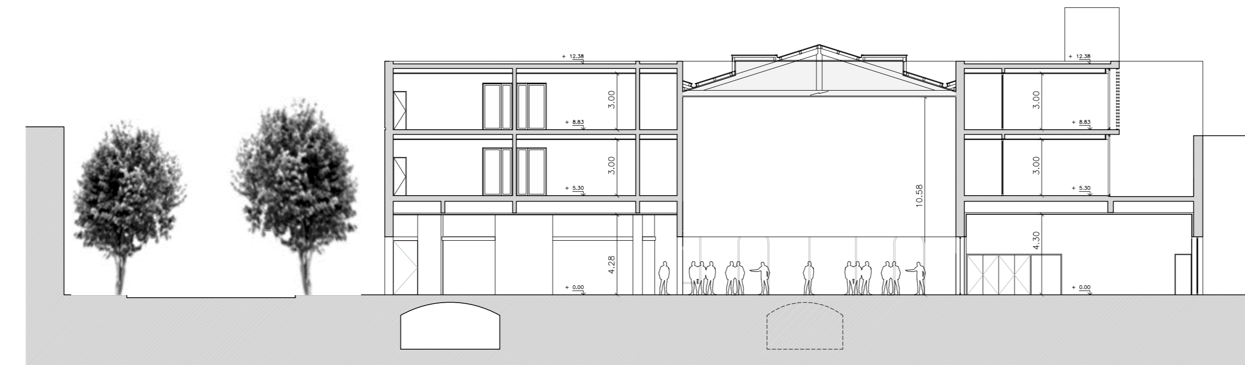
CORTE TRANSVERSAL F-F ESC.:1:200.
